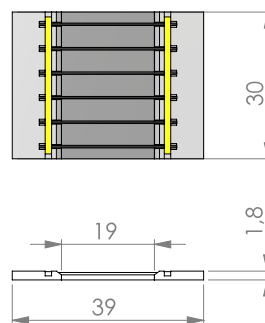
M1930E10 – Actuator Module only
